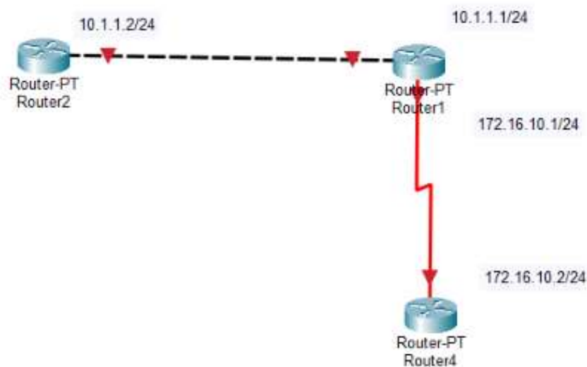
Рисунок 12 – Початкова топологія мережі з неактивними інтерфейсами
